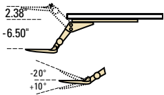
KSFK-21 - 233 $ Mécanisme à profil bas pour tablette à clavier 7,5l x 17,5p x 4,75h
