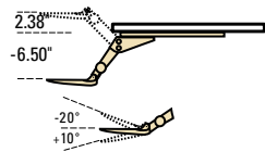
KSFK-21 - 266 $ Mécanisme à profil bas pour tablette à clavier 7,5l x 17,5p x 4,75h
