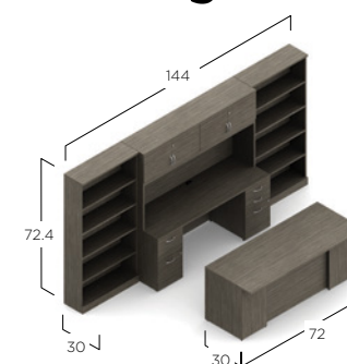
LAYOUT ZIRA EXEC2 Z3072F23+HQ Z2472T Z16L2ES+HQ Z16L2BFS+HQ Z72S42H+HQ ZHBC72 (2) $6935
