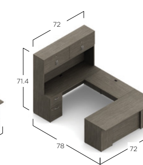
LAYOUT ZIRA EXEC4 Z3072F3R+HQ Z2448FB Z16L2ES+HQ Z2472T Z72S42H+HQ $4497
