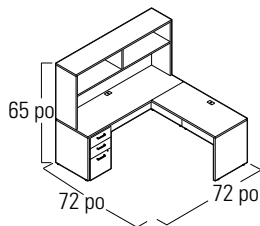
MLP206: Bureau de superviseur avec bahut rectangulaire*
