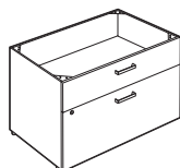
Classeur bas sans dessus, 1 tiroir simple, 1 tiroir classeur
