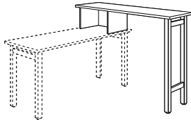
Retour assis-debout
