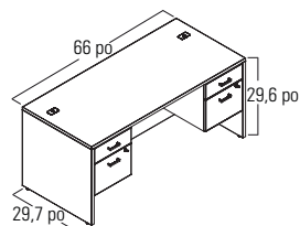
NLP110: Bureau à deux caissons, 66 po x 30 po
