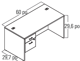
NLP111: Bureau à un caisson 60 po x 30 po*
