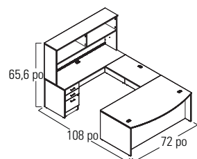
NLP205: Bureau de direction - bureau à devant arqué avec bahut rectangulaire*
