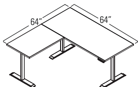
NLP313: Bureau en L à hauteur réglable, 66 po x 66 po* nominale
