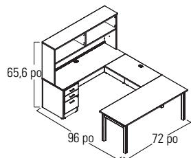
NLP229: Bureau en U*
