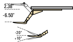
KSFK-21 - 293 $ Mécanisme à profil bas pour tablette à clavier 7,5l x 23,8p x 4,75h
